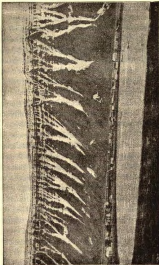
Basaltituntureita isa-vuonosta.
